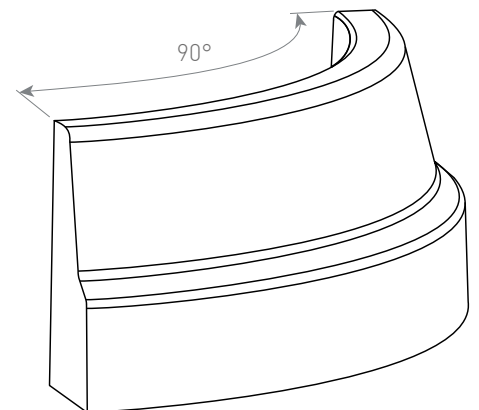
Élément courbe : Rayon : 100 cm Poids : 287 kg
