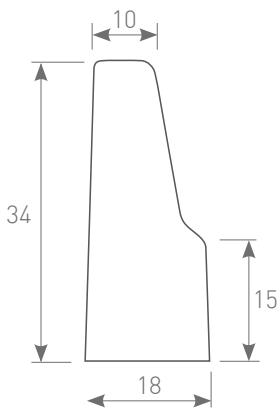
Élément droit : Long. 1m Poids : 75 kg
