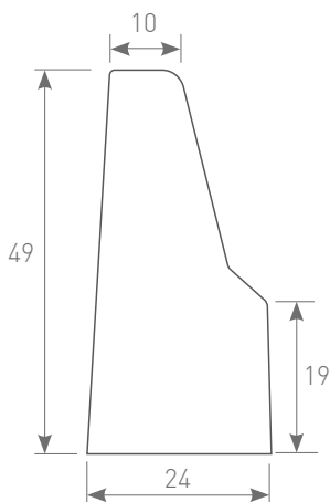
Élément droit : Long. 0,5m - Poids : 107kg Long. 1m - Poids : 215 kg Long. 2m - Poids : 430 kg
